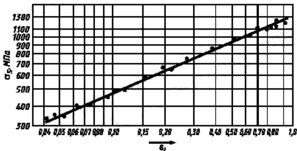
Рисунок 10 — Экспериментальная кривая упрочнения в логарифмических координатах
