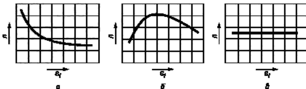
Рисунок Е.1 — Типовые зависимости показателя деформационного упрочнения n от степени деформации \epsilon_j
