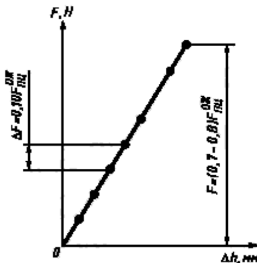
Рисунок 3 — Диаграмма испытаний для определения модуля упругости при сжатии
