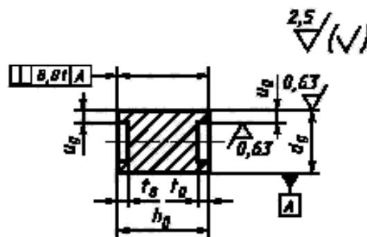
Рисунок 2 — Экспериментальные образцы IV типа
