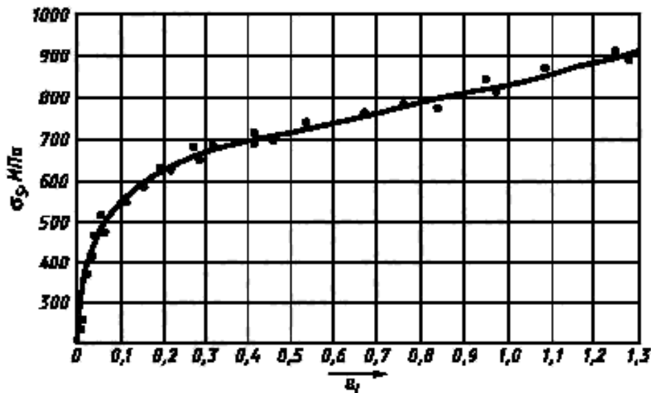
Рисунок 9 — Экспериментальная кривая упрочнения в координатах \sigma_s - \epsilon_l
