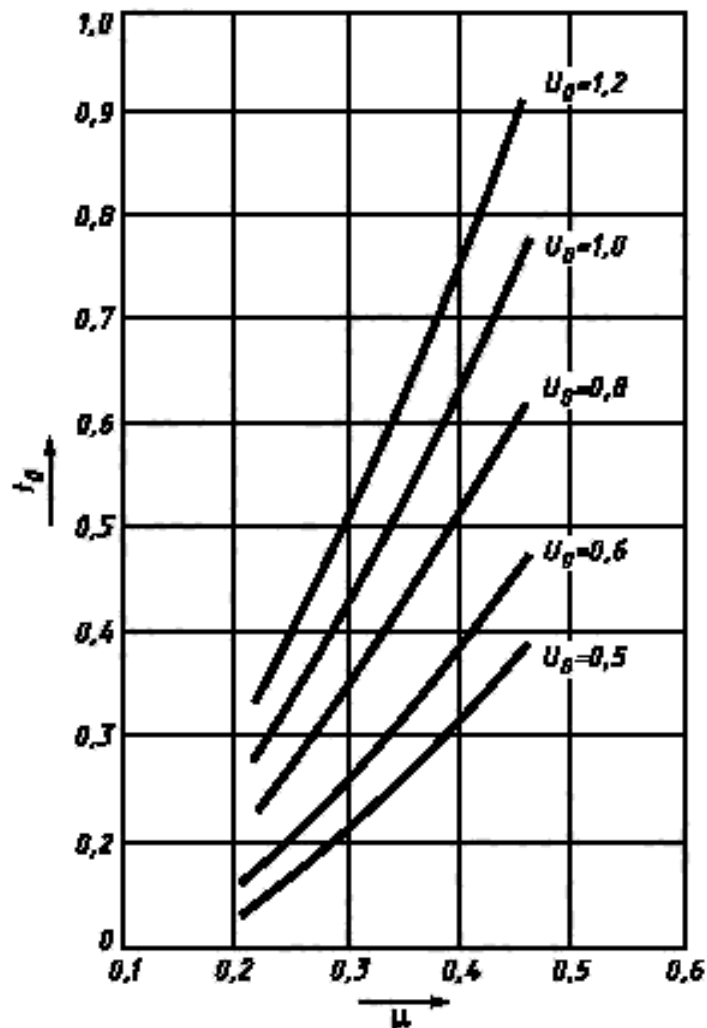
Рисунок А.1 — Зависимость оптимального значения высоты буртиков от коэффициента Пуассона
