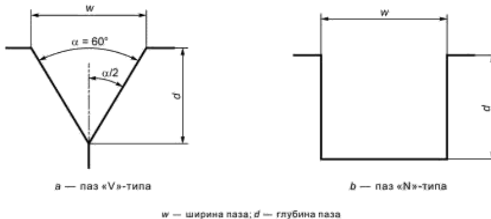
Рисунок 2 — Типы пазов «V» и «N»
